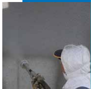
Exemple d'application à la pompe à mortier de Mapelastick sur un viaduc
