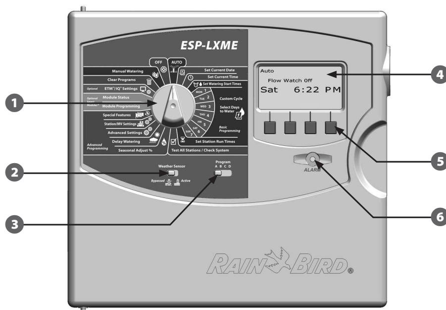
Figure A.1 - Programmeur ESP-LXD - Caractéristiques du tableau de commande
