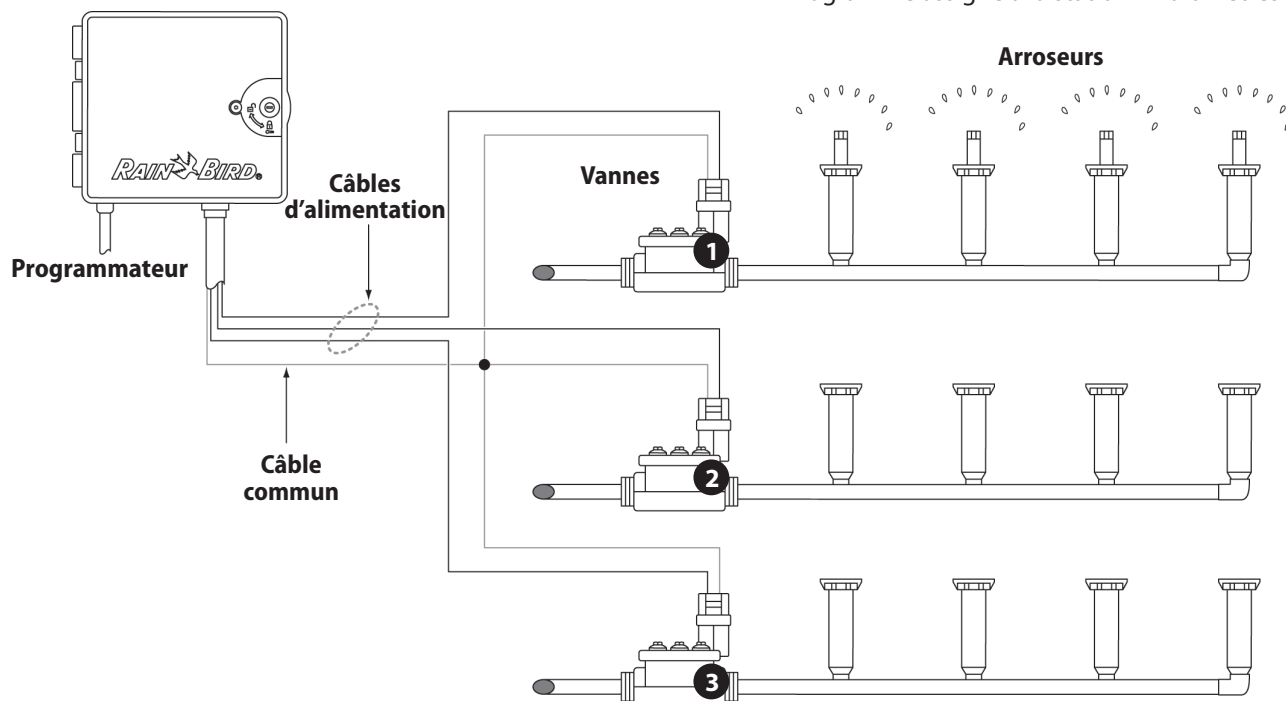
Figure A.2 - Schéma de câblage du système LXME
